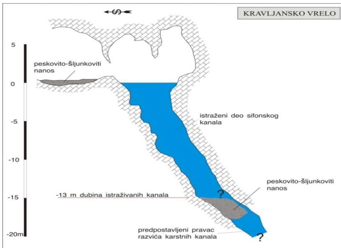
Слика 5: Врело Кравље – профил (Милановић С., 2012)
